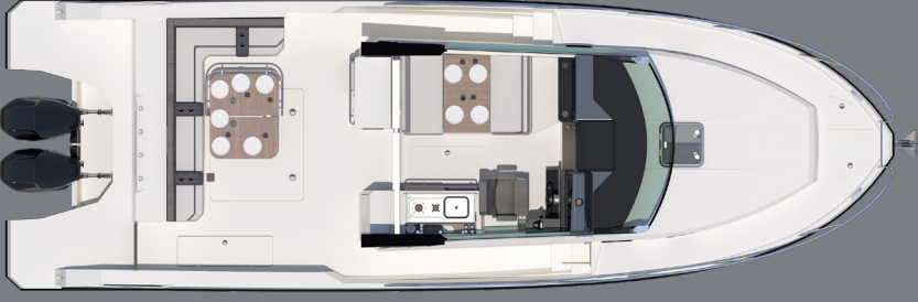
DECK MODULE-2 AND COCKPIT/ GÜVERTE MODÜL-2 VE KOKPİT
